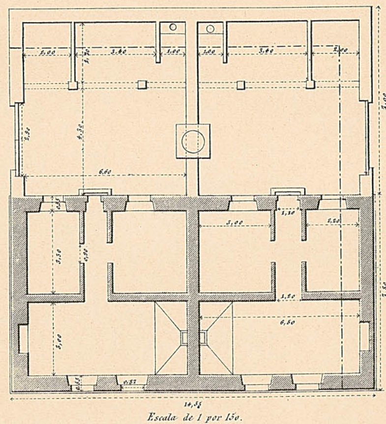
Fig. 64 a Planta del modelo del Sr. Boquerin.
