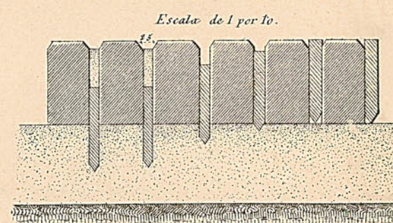
Fig. 55 a Entarugado sobre arena.
