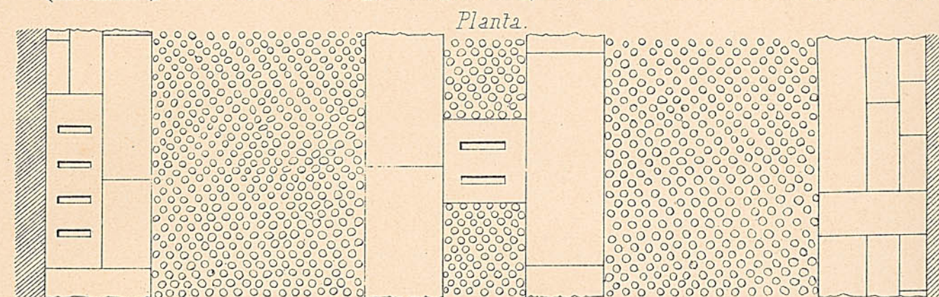
Fig. 56 a Entarugado sobre hormigón.
