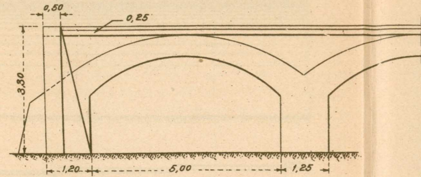
PONTON MODELO N° 4.
