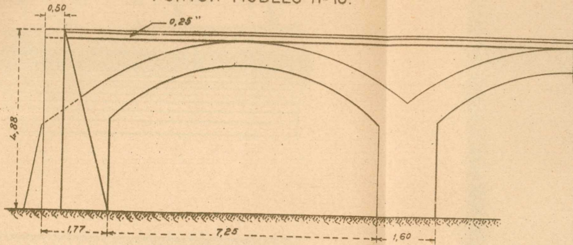
PONTÓN MODELO Nº 10.
