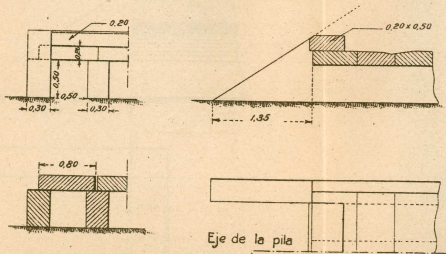
TAJEA MODELO Nº 1
