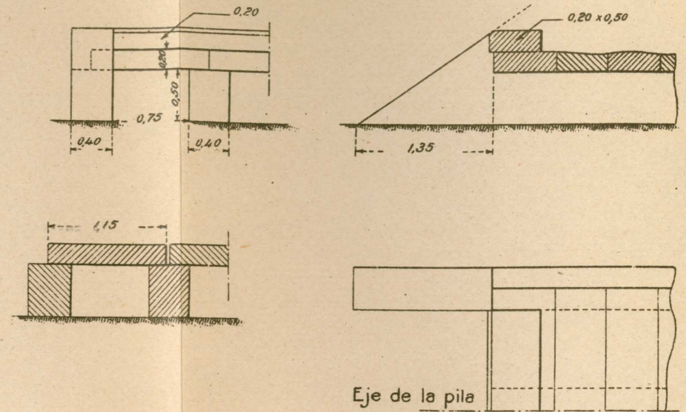
TAJEA MODELO Nº 2
