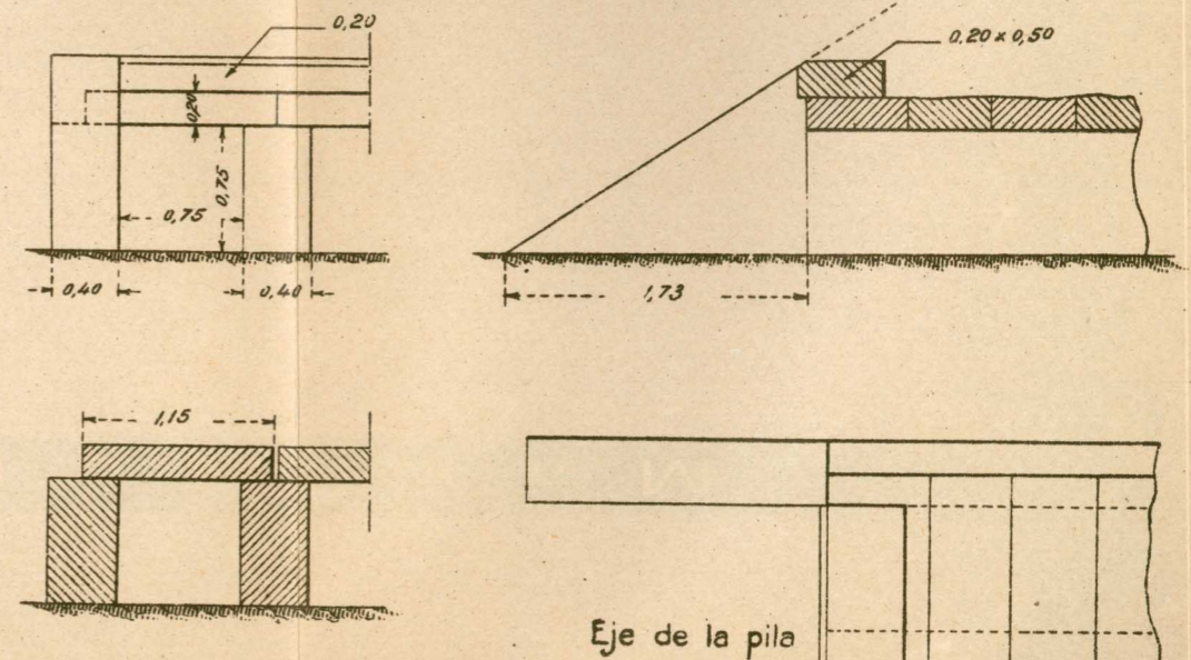
TAJEA MODELO Nº 3
