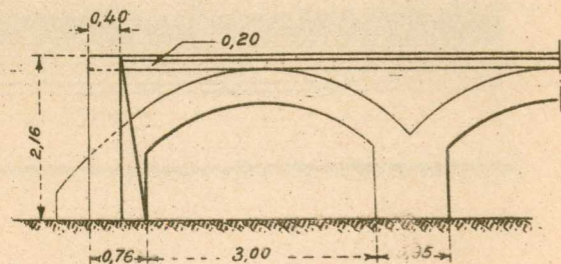
ALCANTARILLA MODELO Nº 3
